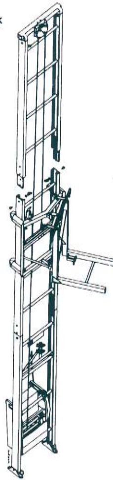
Senkrecht mit Schubkarrenbühne und -schlitten bis 60 Meter (nur Geda)
