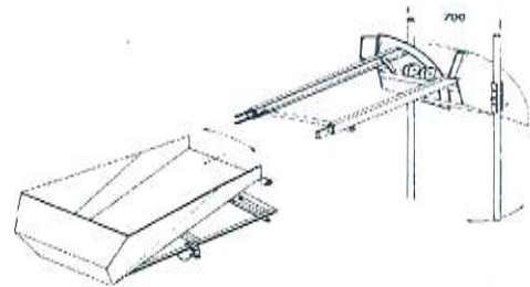
Kippmulde für Standardschlitten (Geda)
