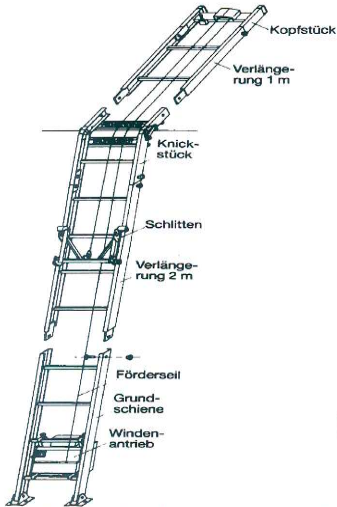
Schräg mit Knickstück und montierter Dachverlängerung bis 20 Meter (Pauss und Geda)
